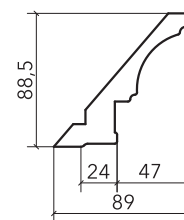
VD122 карниз верхний из МДФ с накаткой из древесной пасты L= 3700 мм
